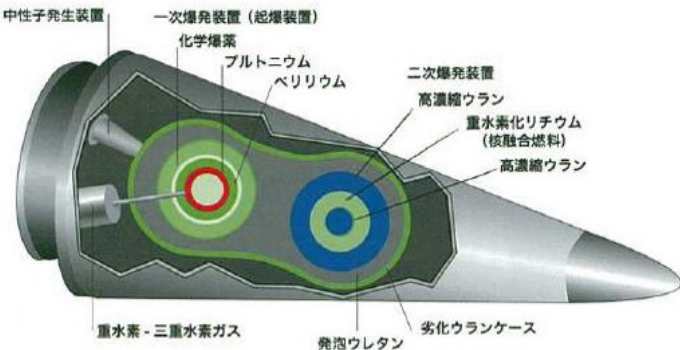
一般的な核弾頭の概念図
